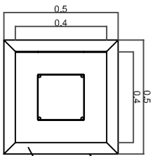
PROYECCION DE LA BASE DE CONCRETO ENTERADA A 0.60 MTS
