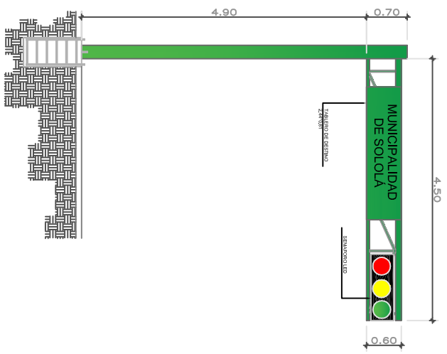
ELEVACION FRONTAL
